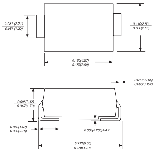
SMA/DO-214AC
